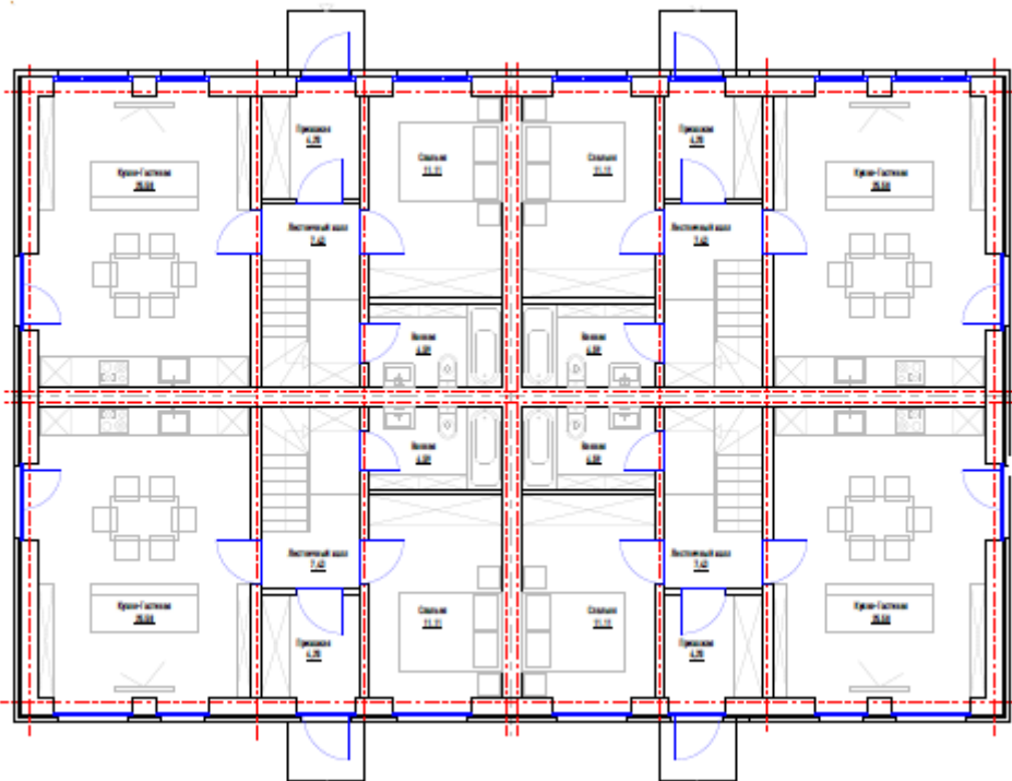
План 1 этажа
