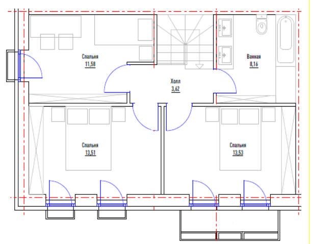
План 2 этажа
