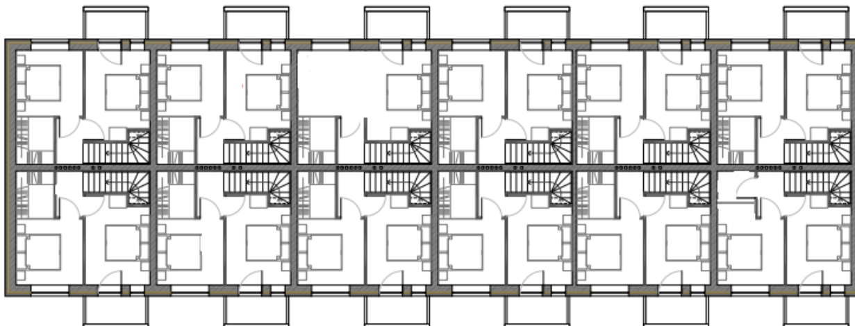
План 2 этажа
