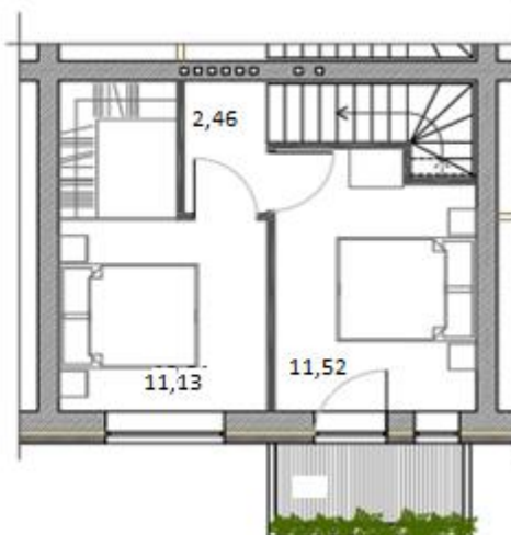
План 2 этажа
