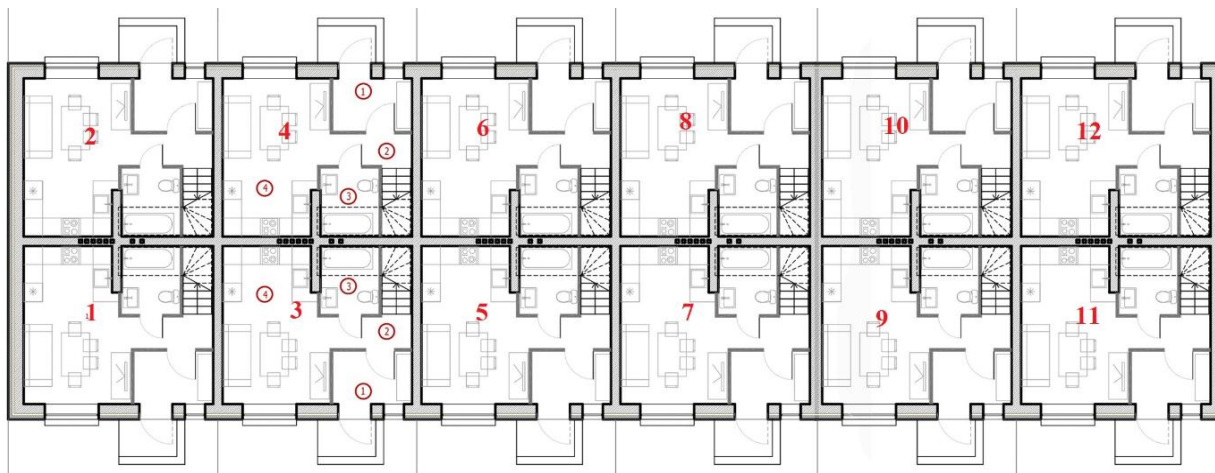
План 1 этажа
