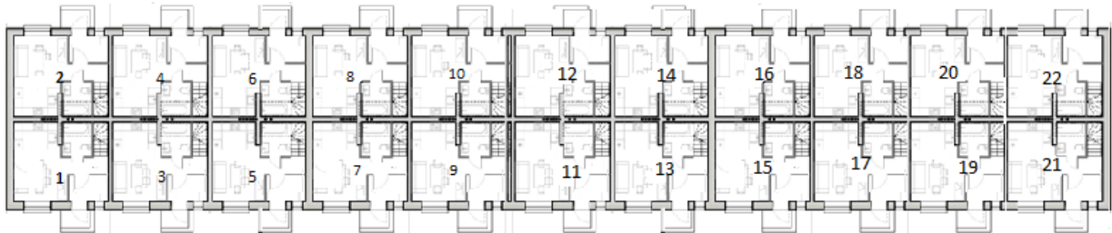
План 2 этажа
